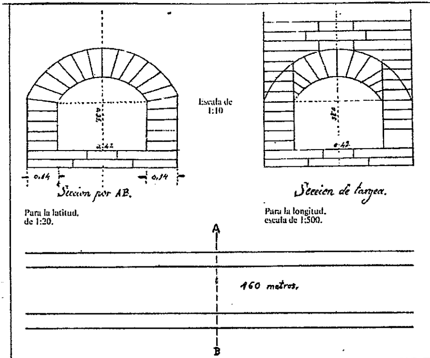
Proyecto de una targa de desagüe en el lavadero público de la villa de Getafe año 1888.
